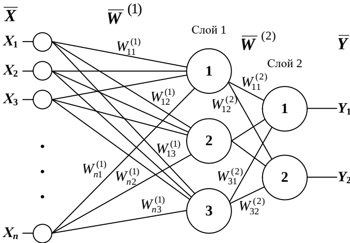
Рис. 25. Двухслойный перцептрон
