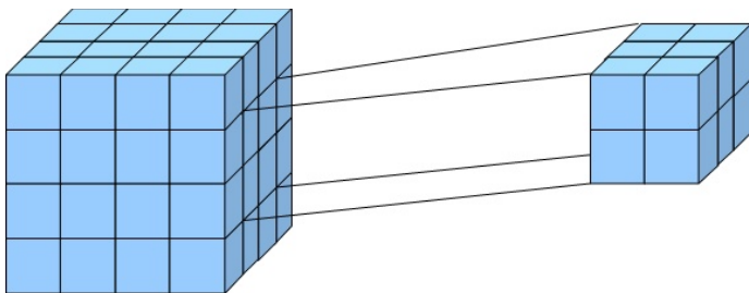
Рис. 4. Операции OLAP: детализация
