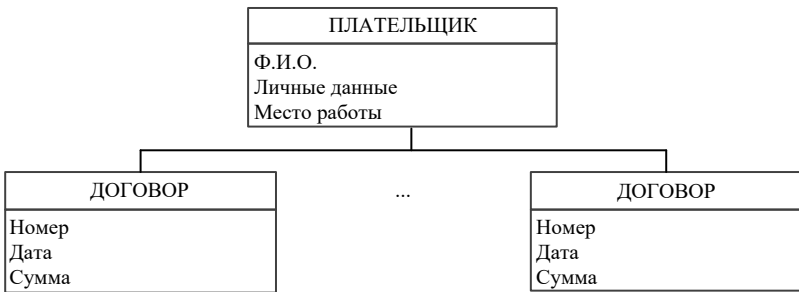
Рис. 16. Дополнительное групповое отношение студент — договор — плательщик
