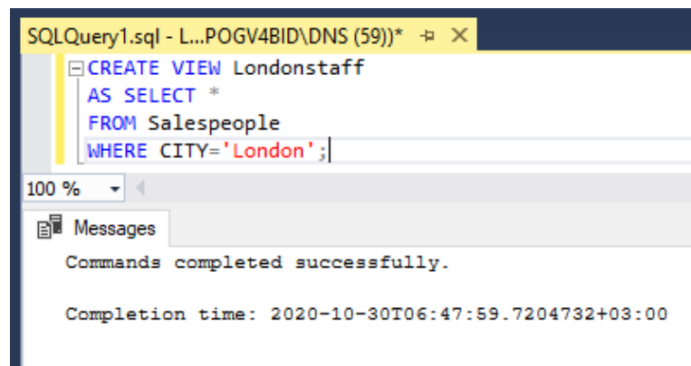
Рис.65. Создание представления Londonstaff
