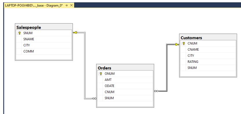
Рис. 21. Диаграмма базы данных Training_base
