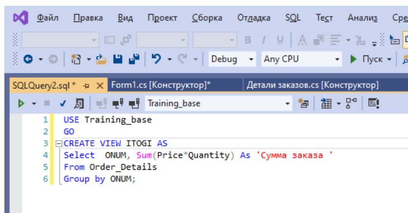
Рис. 117. Создание представления ITOGI
