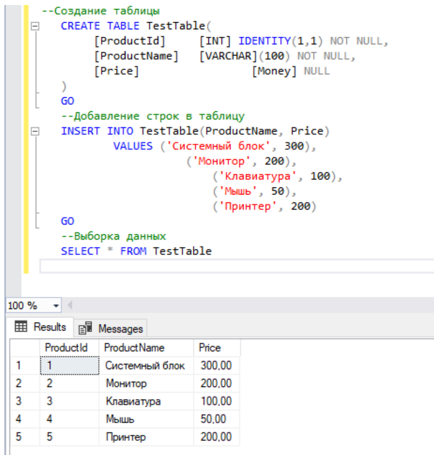
Рис. 55. Создание таблицы с данными
