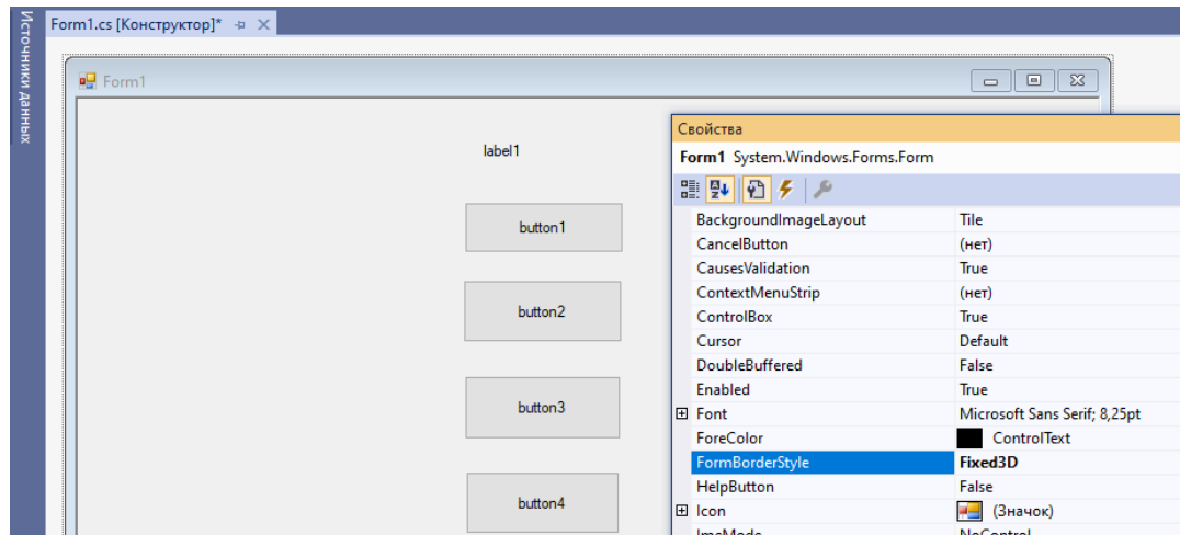
Рис. 88. Параметры свойств формы
