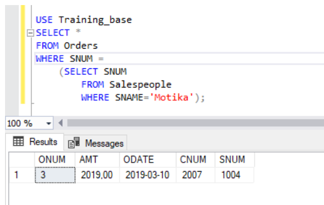
Рис. 51. Окно выполнения запроса 19
