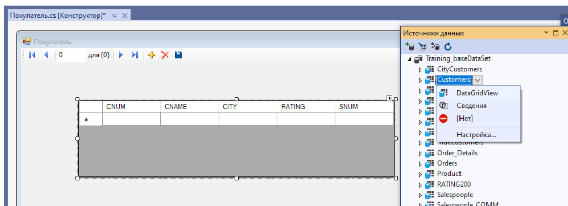
Рис. 96. Внешний вид формы с таблицей, опирающейся на информацию из источника данных
