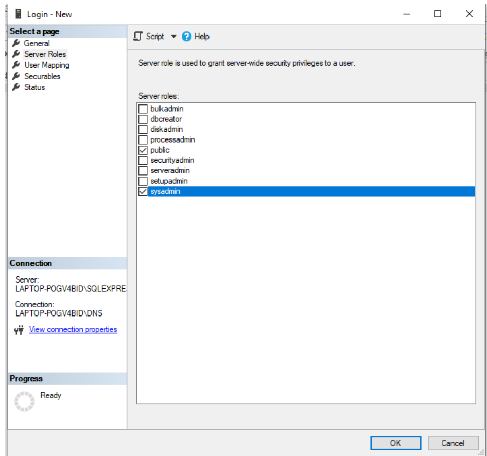
Рис. 73. Настройка серверной роли для нового пользователя
