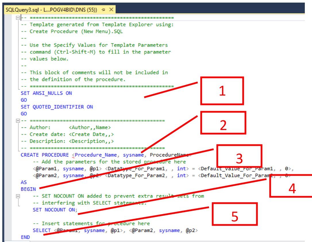
Рис. 66. Окно новой хранимой процедуры
