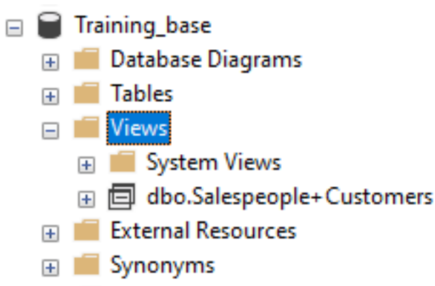
Рис.61. Отображение нового представления в обозревателе объектов
