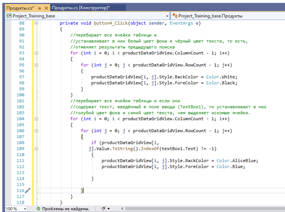
Рис. 114. Код обработки события нажатия кнопки Найти
