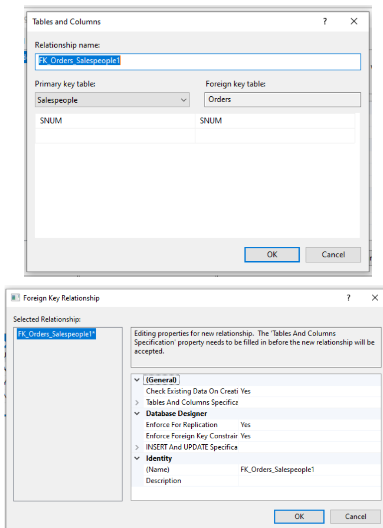
Рис. 20. Установление связи между таблицами
