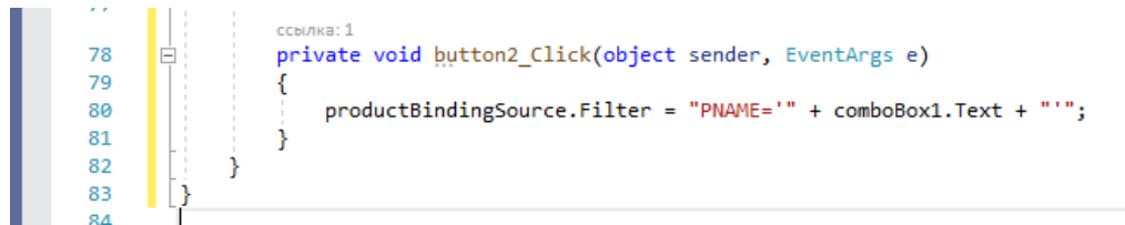
Рис. 112. Код обработки события нажатия кнопки Фильтровать
