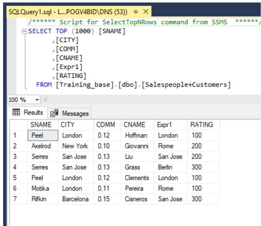
Рис. 62. Выполнение запроса Salespeople+Customers
