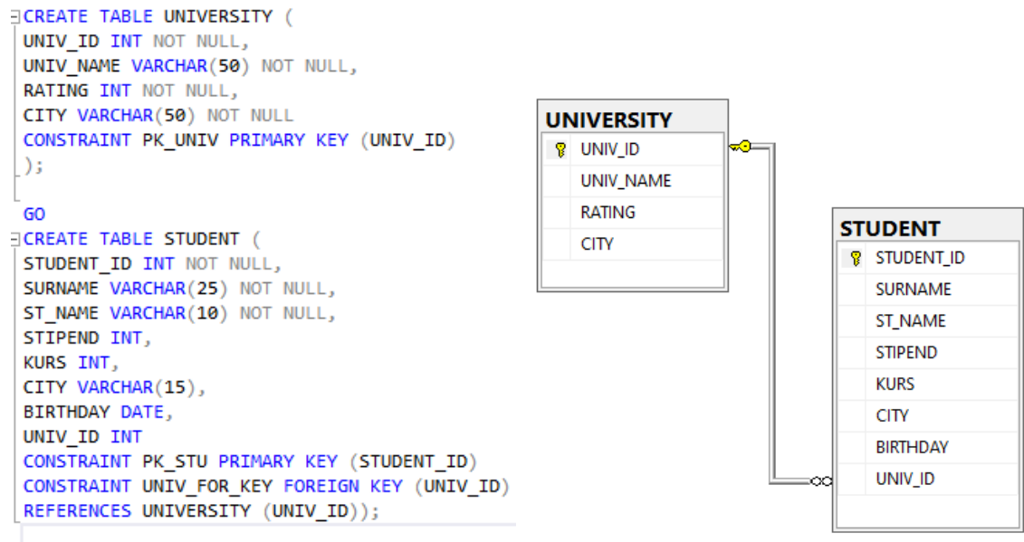
Рис. 21.1. Создание связи с помощью конструкции FOREIGN KEY
