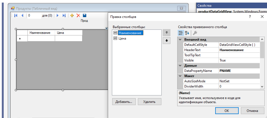
Рис. 108. Окно Правка столбцов
