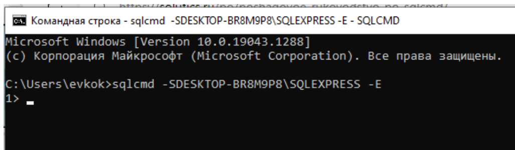
Рис. 70.2. Подключение к серверу
