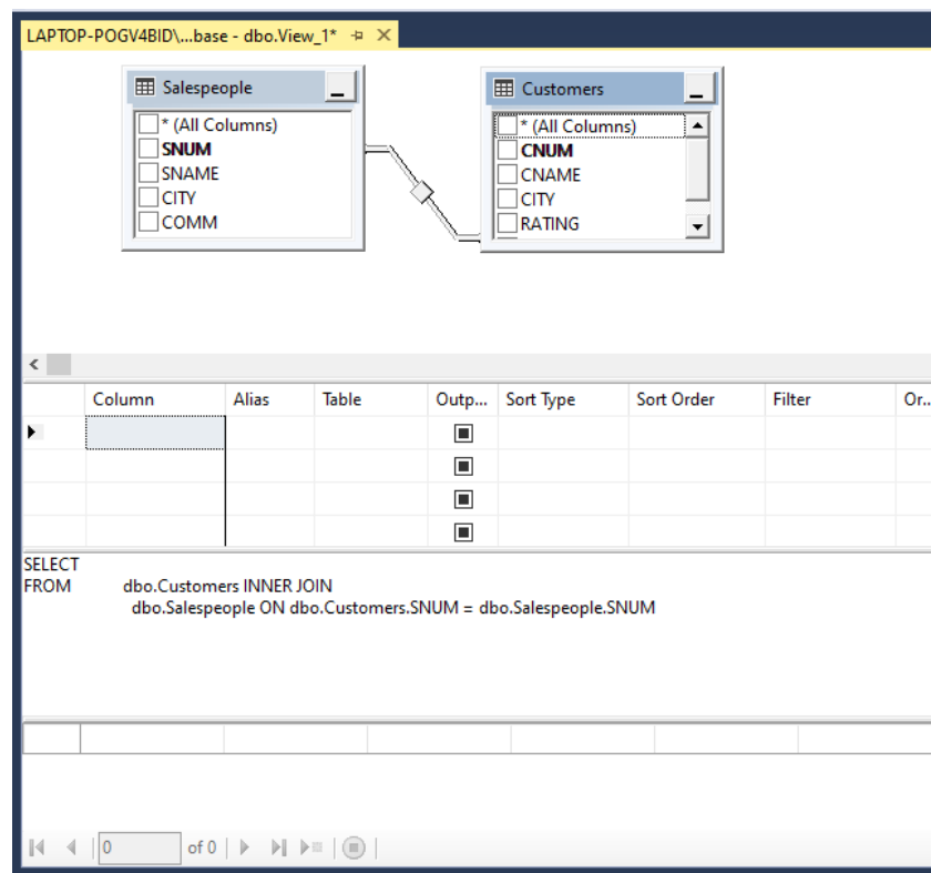
Рис. 59. Окно конструктора запросов
