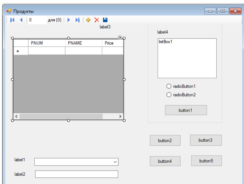
Рис. 106. Добавление таблицы Product на форму
