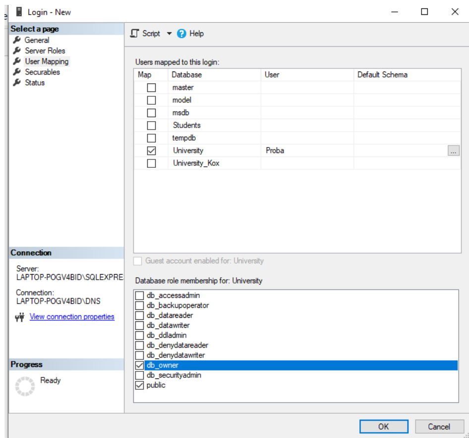
Рис. 74. Настройка роли базы данных для нового пользователя
