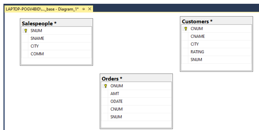
Рис. 19. Добавленные таблицы на диаграмму
