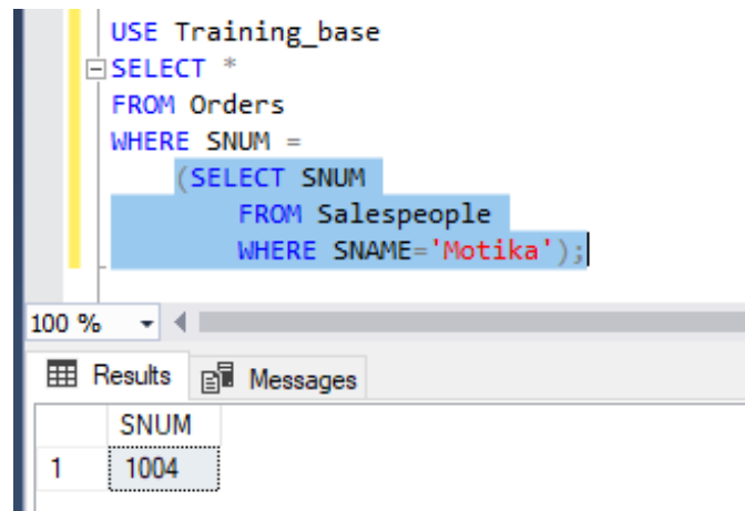
Рис. 50. Окно выполнения подзапроса
