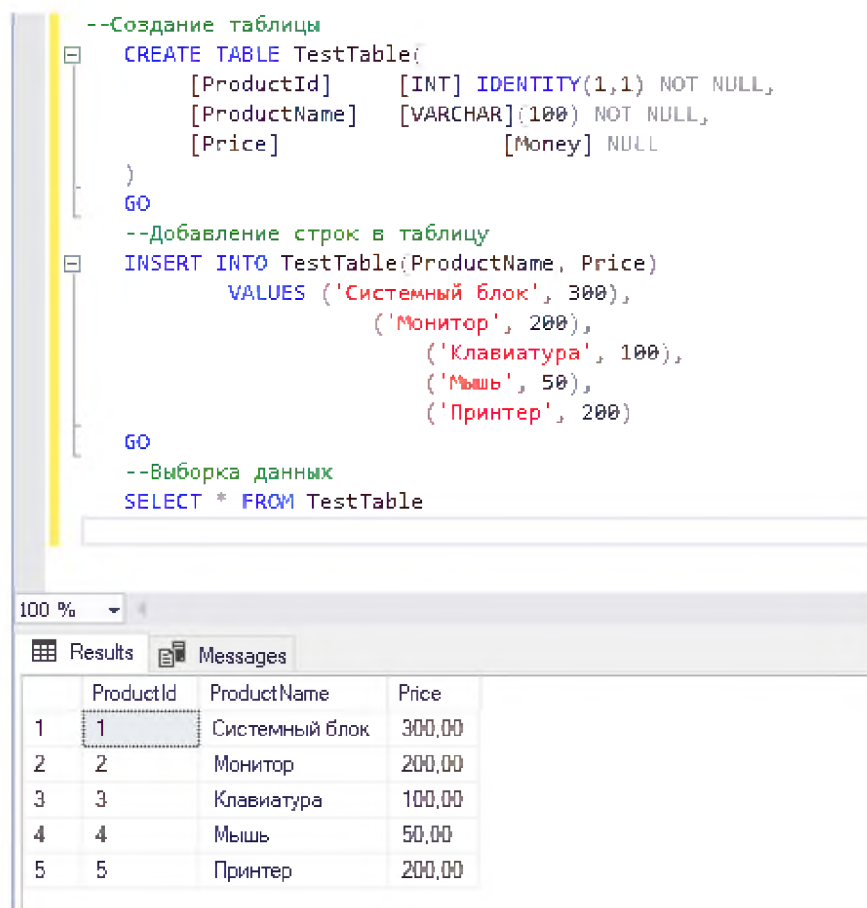
Рис. 55. Создание таблицы с данными
