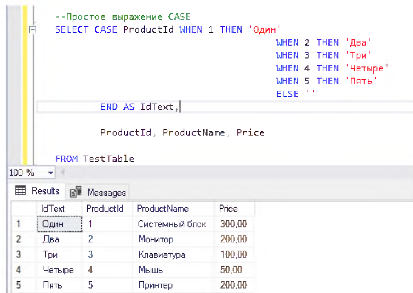
Рис. 56. Пример простого выражения CASE в инструкции SELECT
