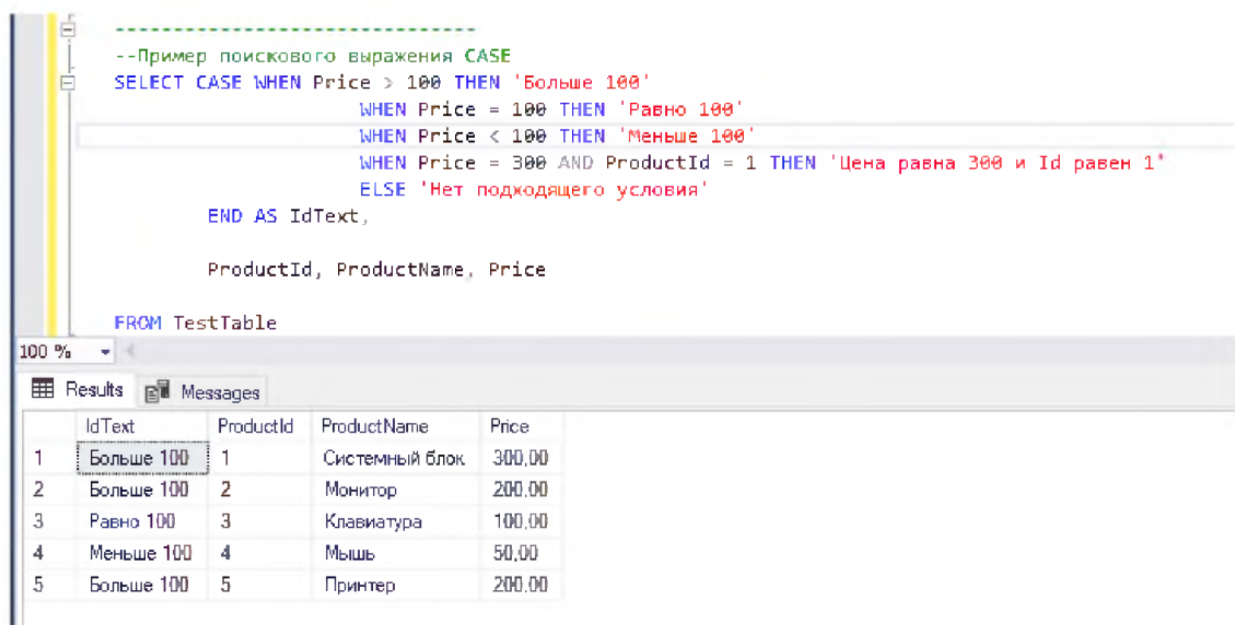
Рис. 57. Пример поискового выражения CASE в инструкции SELECT
