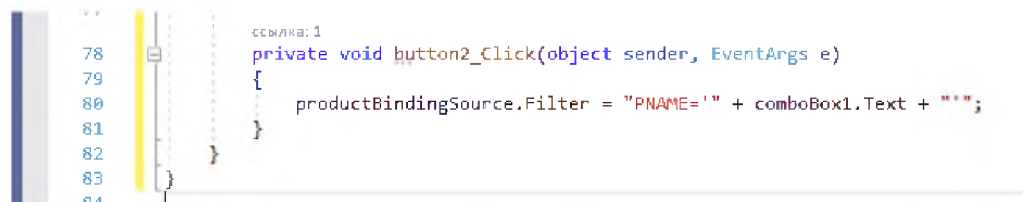
Рис. 112. Код обработки события нажатия кнопки Фильтровать
