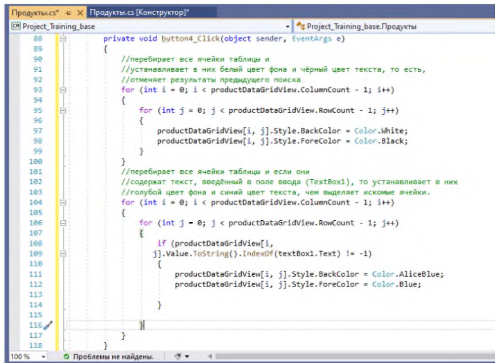
Рис. 114. Код обработки события нажатия кнопки Найти
